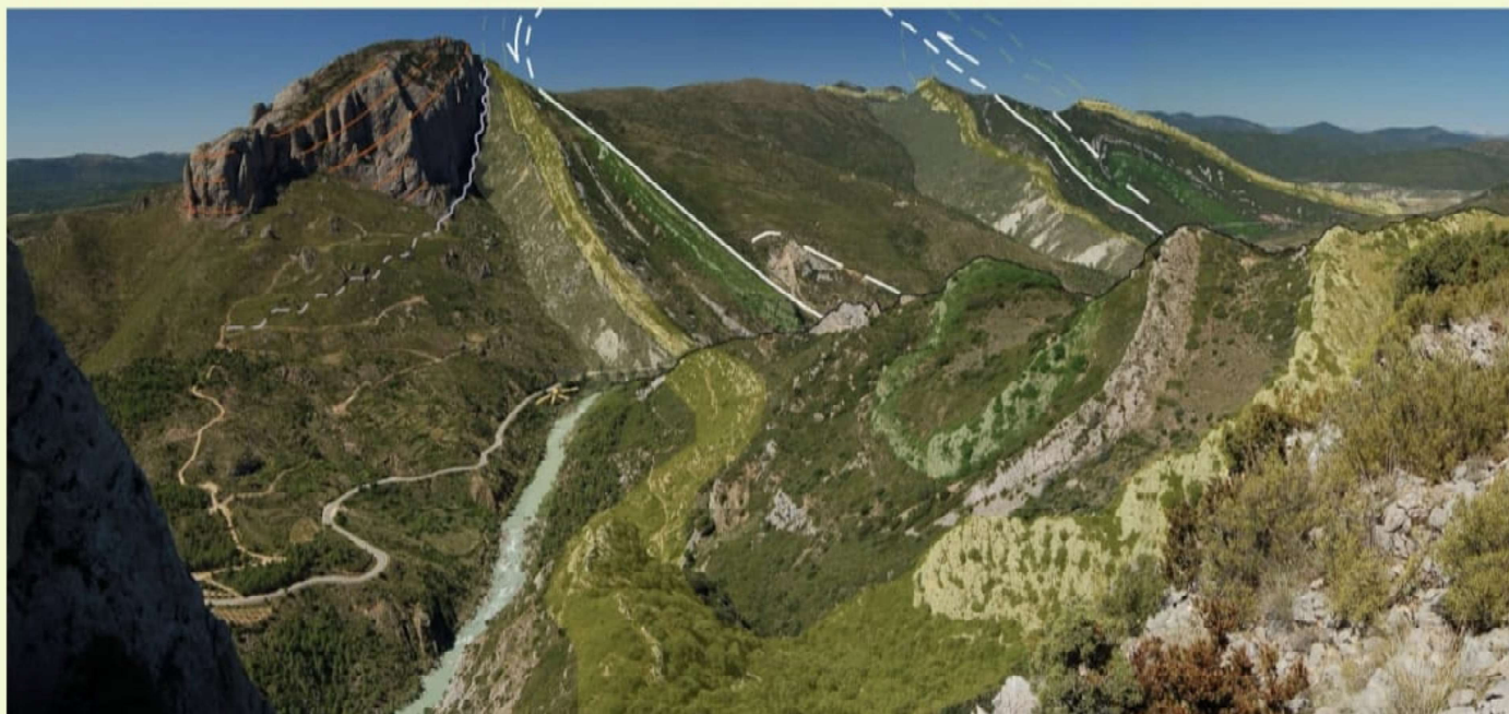
Esbozo de interpretación geológica del corte del río Gállego entre Peña Rueba -en la imagen- y los Mallos de Riglos (Foto: J.L.Piedrafita)
