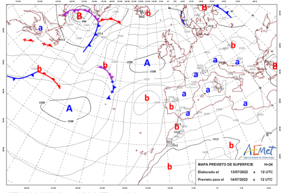
Mapa de superficie 14/07/2022 14:00 h
