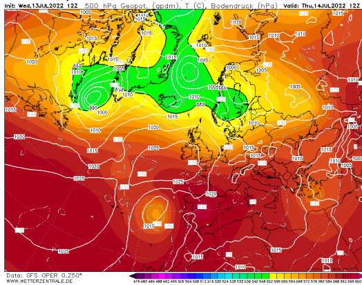
Mapa de 500 hPa 14/07/2022 12 UTC GFS
