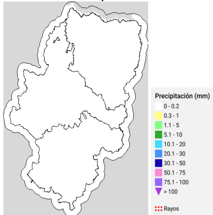
Precipitación
