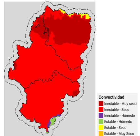
Convectividad 17h
