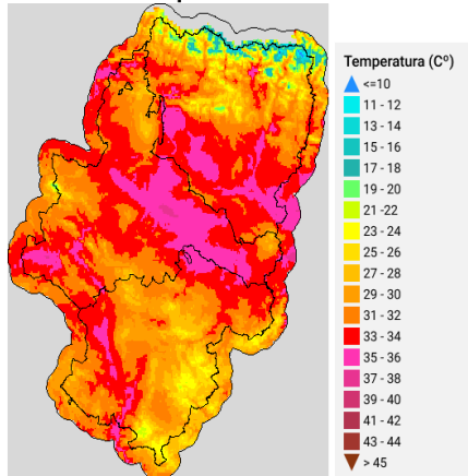
Temperatura máxima
