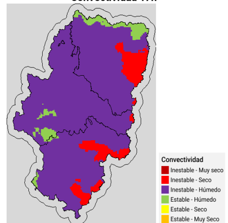
Convectividad 17h
